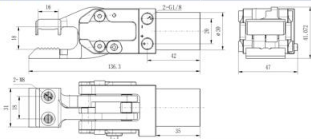
未安装钳头示意图
