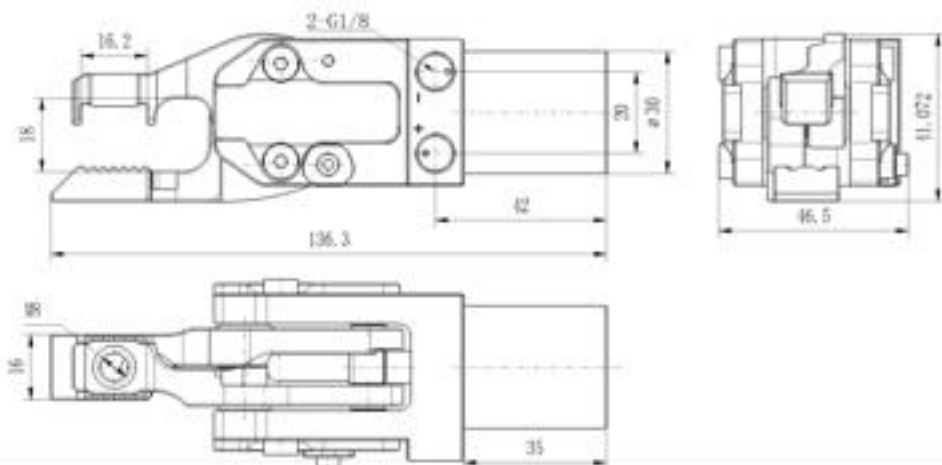
未安装钳头示意图
