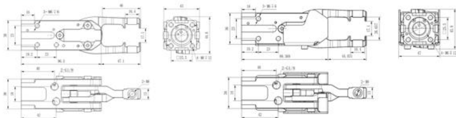
夹钳钳头示意图
