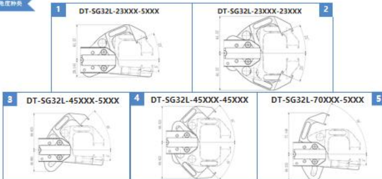
夹钳打开角度种类
